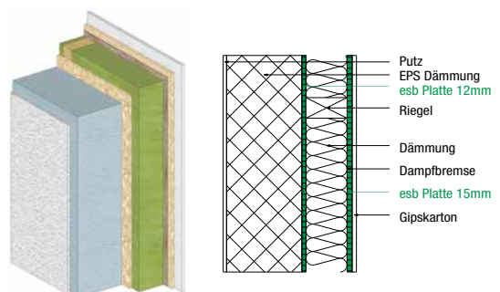
Außenwand 4 – mit Wärmeverbundsystem EPS
