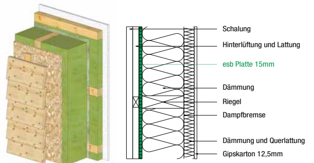
Außenwand 2 – hinterlüftet
